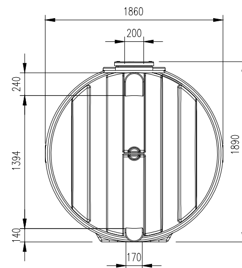
VISTA LATERAL DIREITA
