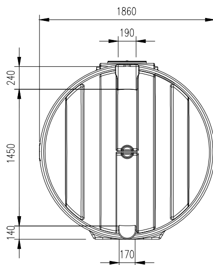
VISTA LATERAL ESQUERDA
