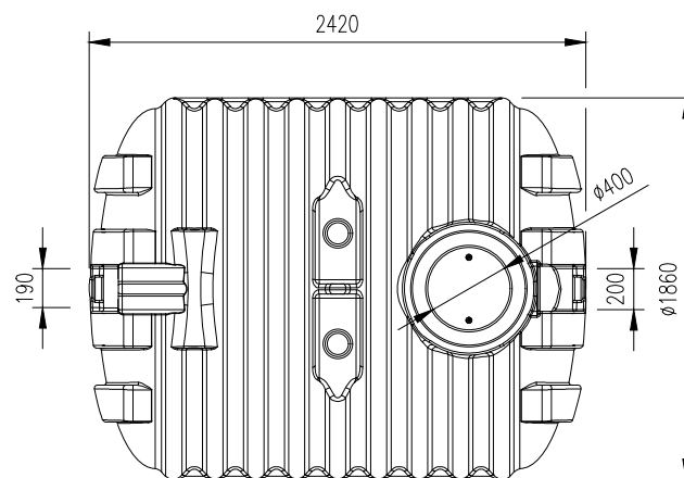
PLANTA
