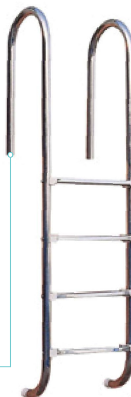
A - Escada de muro inclui ancoragem com ligação terra (AISI 316L)
