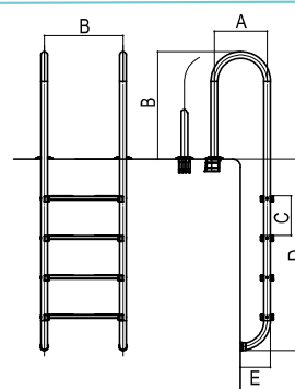
A - Escada de muro inclui ancoragem com ligação terra (AISI 316L)
